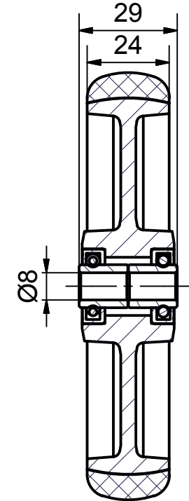
SECTION A-A'
