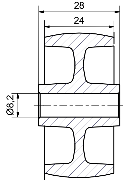
SECTION A-A'
